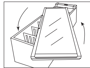
3. Skleněné dveře obraťte (u FZ 295 W stáhněte rukojeť tak, že se uvolní zevnitř pod těsnicí lištou).
