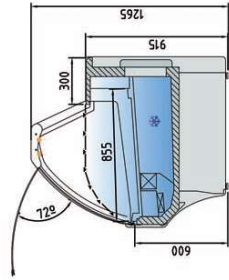
VE-10E-C-TF
