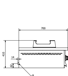
OPCIÓN QUEMADOR WOK 18kw WOK BURNER GAS CIRCUIT 18kw
