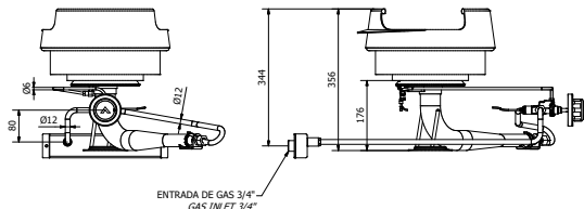
OPCIÓN QUEMADOR WOK 18kw WOK BURNER GAS CIRCUIT 18kw
